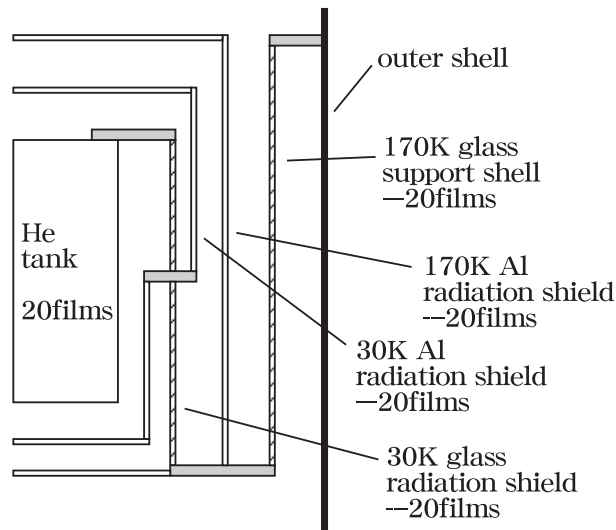
図 3.2: 熱制御フィルムの巻いている箇所
