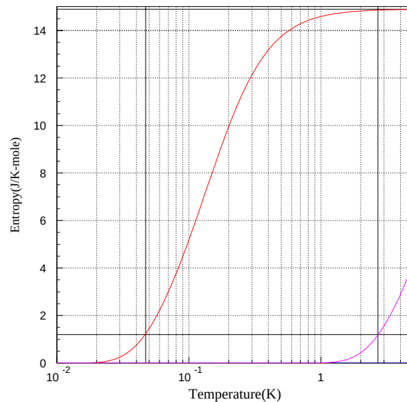
図 4.12: 内部磁場を 600Gauss とした時の温度 — エントロピー曲線。紫が最大磁場。赤は内部磁場のみの場合。
