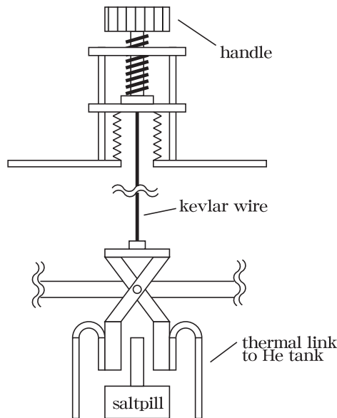
図 3.14: メカニカルヒートスイッチの構造図
