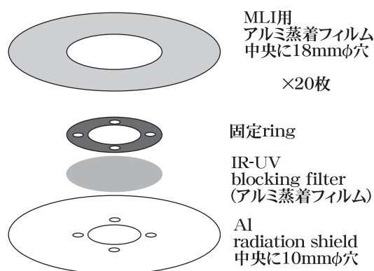
図 6.7: 導入した入射窓の構造図。実質の入射窓の大きさは 10mmφ。
