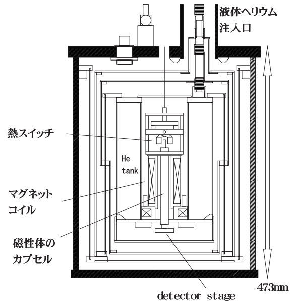
図 2.8: ADR デュワーの構造図。
