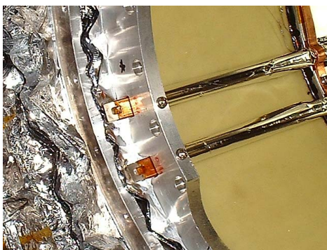
図 3.12: HE tank サポートリングにとりつけた高温超伝導リード線。手前が cold end cap。
