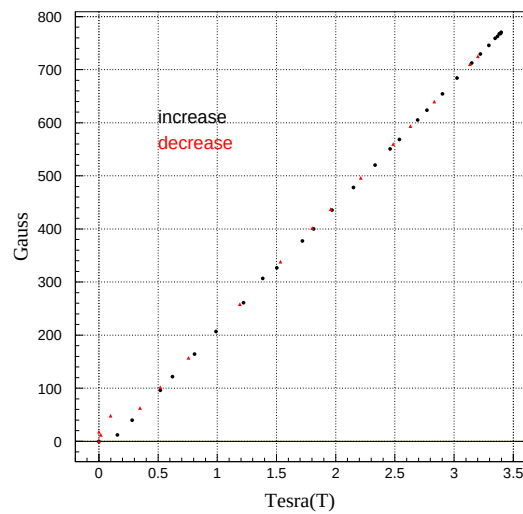
図 7.10: 02/07/07 におこなった SQUID 導入部分の磁場測定結果
