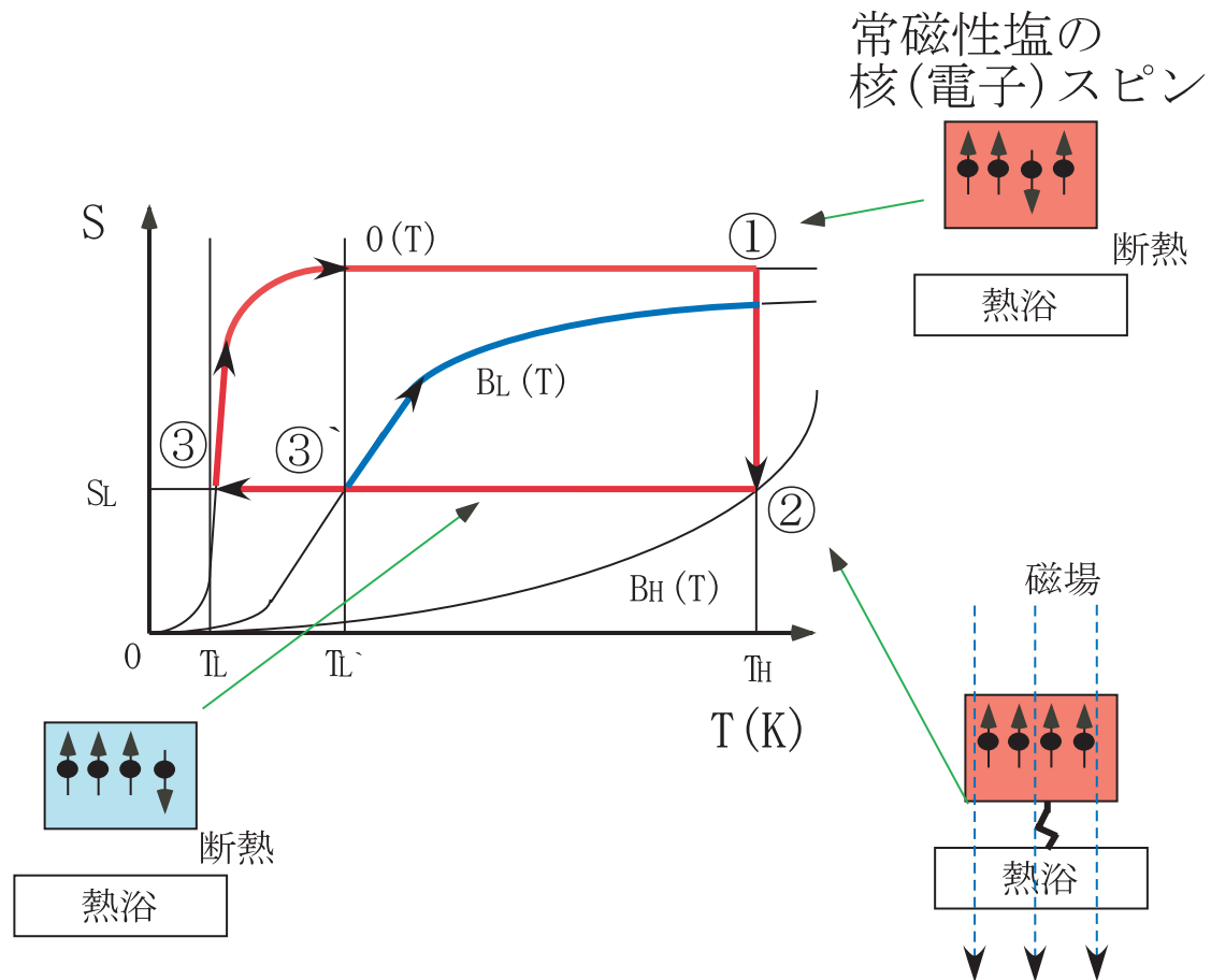
図 2.2: 冷却課程でのエントロピーと温度の関係グラフ
