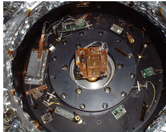
図 8.2: TES 型マイクロカロリメータ導入図。
