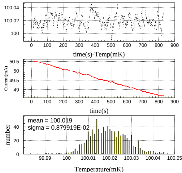
図 5.7: DISPLAY-Tc=8s で制御させた際の結果。rms=8.8 \mu K。
