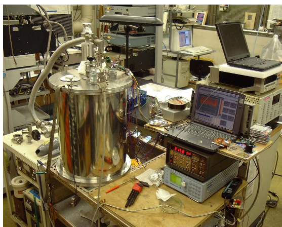
図 4.2: ADR 冷却試験時のデュワー図。右側の装置は温度モニター用 PC など。
