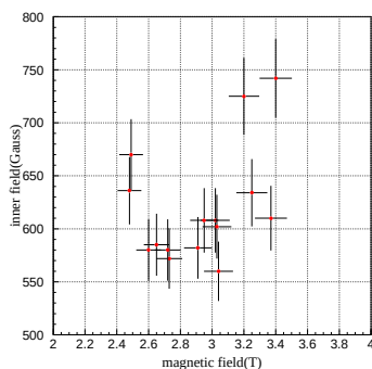
図 4.9: 断熱消磁試験結果の最大磁場と内部磁場の関係。
