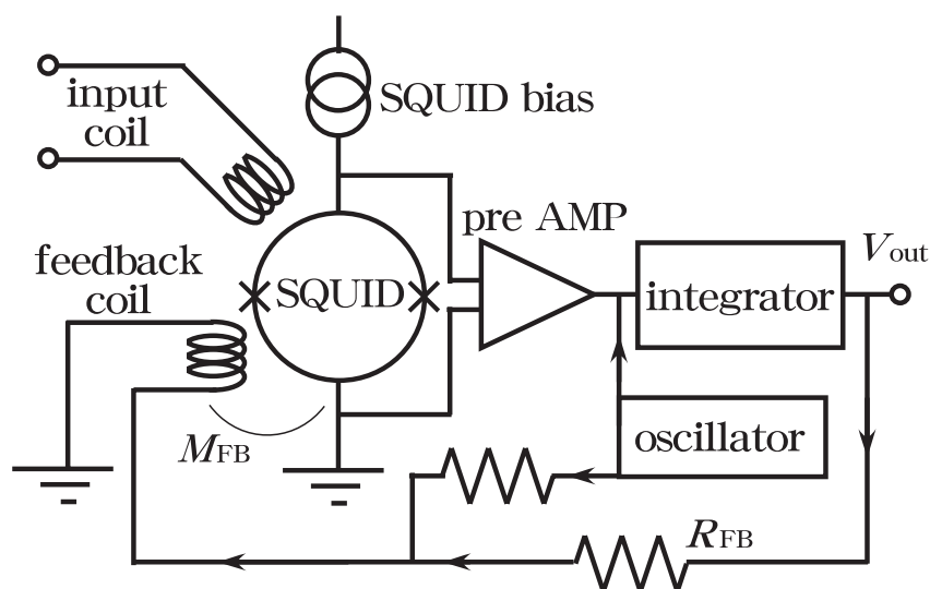
図 7.4: Flux Locked Loop. FLL のフィードバック機構
