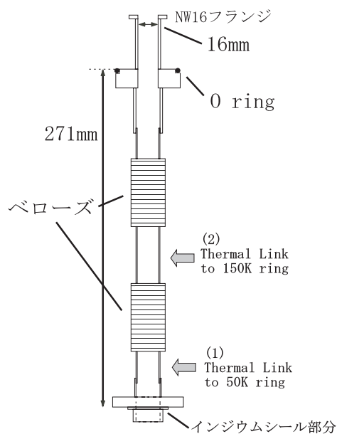
図 3.4: Vapor Cooling System 用タワー
