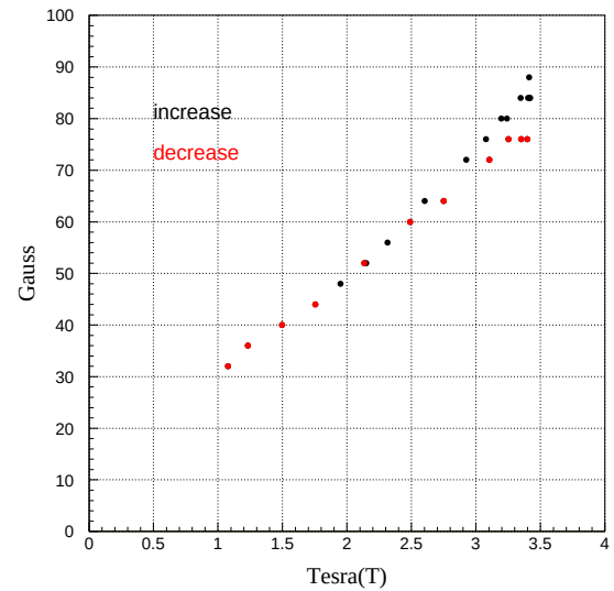
図 7.9: 02/05/15 に行なった detector table 周辺の磁場測定結果。黒 : magnetization、赤 : demagnetization
