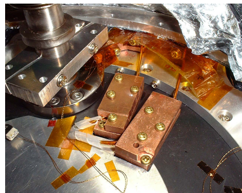
図 3.13: cold end cap の熱リンクの図。NbTi 線を He tank と熱リンクをとった銅部品ではさんでいる。
