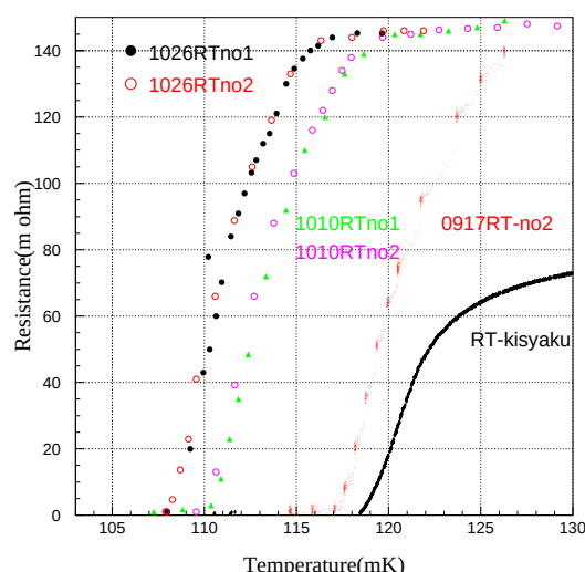
図 6.11: 入射窓導入による RT 測定の変化。導入によって遷移温度が 10mK 程度変化している。2 日とも 2 回の測定でほぼ同一直線上。
