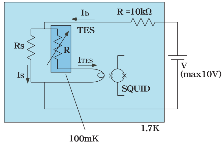
図 8.3: TES マイクロカロリメータを動作させるための回路図
