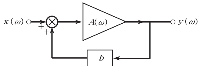
図 7.3: フィードバック回路図
