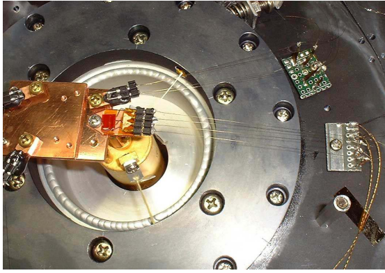
図 7.8: 極低温部に導入したホール素子。極低温部に 3mm 厚の銅板をのせ、温度計 2 つ、さらにヒーターと同時に導入している。
