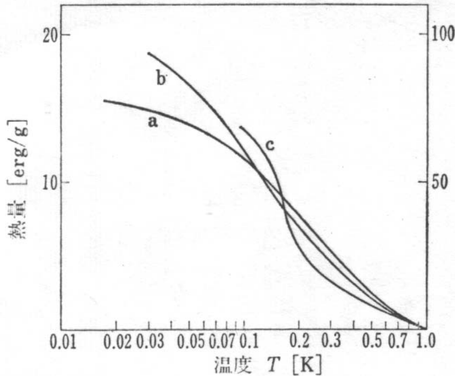
図 2.1: 常磁性塩の、 1 \text{ K} まであげるのに要する熱量 (erg/g) ([16] より)。a: CrK ミョウバン b: Fe(NH 4 ) ミョウバン c: Mn(NH 4 ) Tutton 塩
