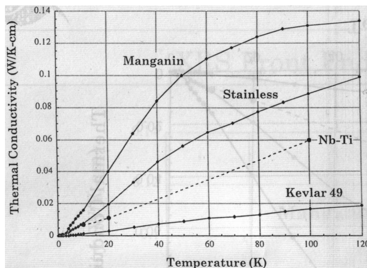
図 3.7: マンガン線の熱伝導率の温度特性 ([25] より)
