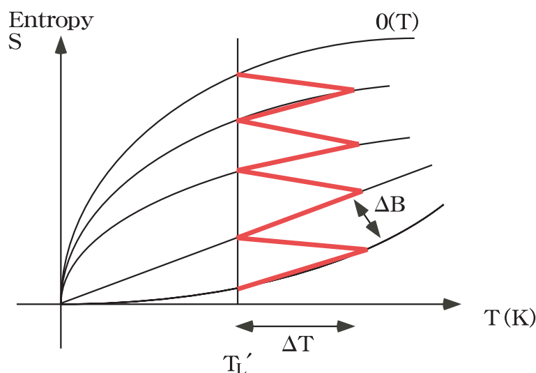
図 2.3: 温度制御の原理
