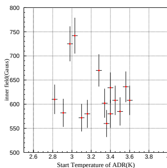
図 4.10: 断熱消磁試験結果の消磁開始温度と内部磁場の関係。
