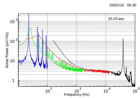
図 7.17: ノイズパワースペクトル。02/12/30.
