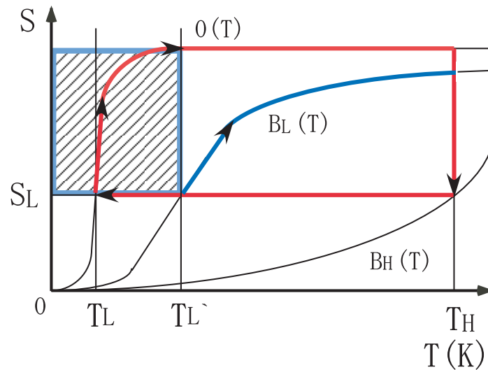
図 6.12: 断熱消磁冷凍機の、等温にした場合の熱容量。図の斜線部分。
