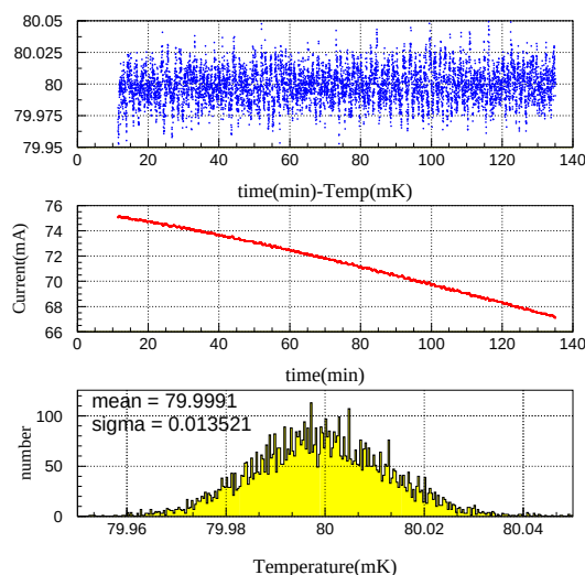
図 5.6: 2 時間制御させた際の結果。rms=13.6 \mu K。
