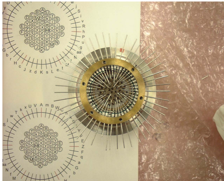
図 3.8: 直線タイプ、 \pi 型 EMI フィルタをとりつけたコネクタ. feed through には KYOCERA 48PINtype を使用. 写真は裏側 (高真空側).
