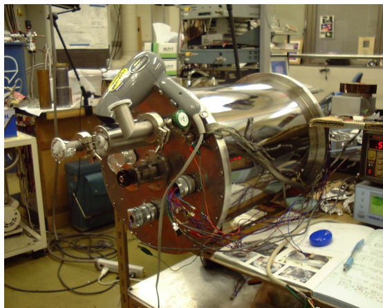
図 4.18: ヘリウム注入後、横に倒した状態の ADR デュワー
