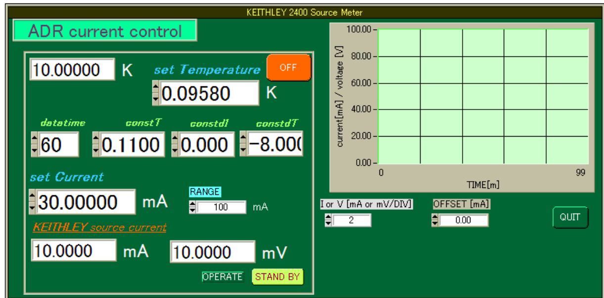
図 5.3: k2400 panel(Lab Windows)
