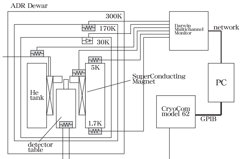
図 3.9: 温度計の取り付け箇所と配線系統
