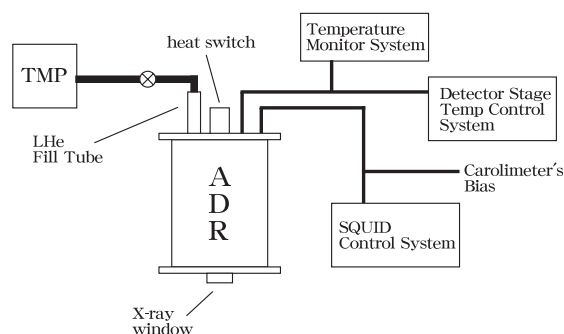
図 4.3: 冷却実験の装置の配置図
