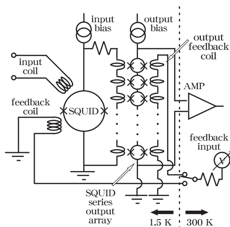
図 7.5: TSS AMP の回路図
