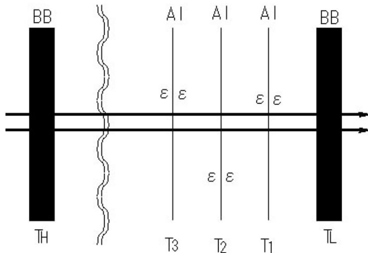
図 3.1: 黒体間においたアルミのフィルム
