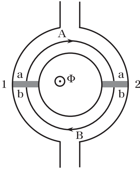
図 7.1: dc-SQUID 素子の模式図
