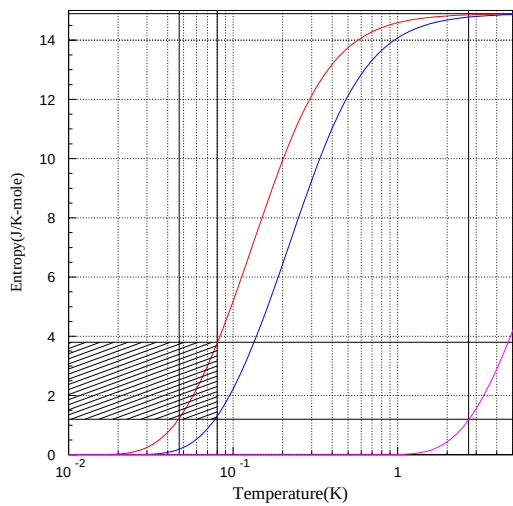
図 6.13: 典型的な冷凍サイクルでのエントロピー曲線。
