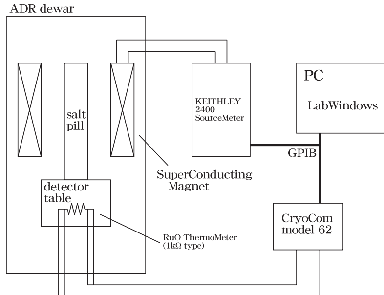
図 5.1: 温度制御の構成図
