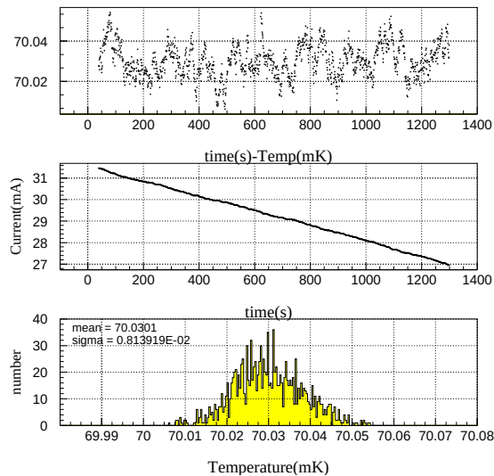
図 8.1: 03/01/20 に行なった温度制御結果。 \text{rms}=8.14\mu\text{K} 。
