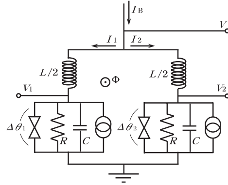
図 7.2: dc-SQUID 素子の等価回路
