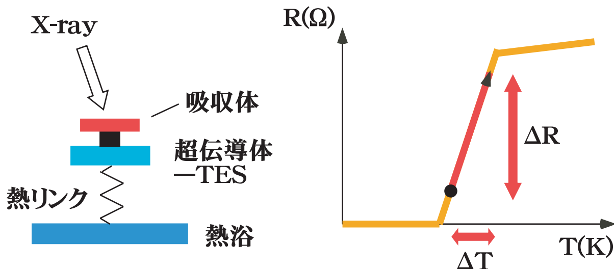
図 1.3: TES 型マイクロカロリメータの動作概略。吸収体に X 線が入射するとそのエネルギーに伴って温度上昇する。これを TES が捕え、TES の抵抗が増す。温度変化に対して抵抗変化の大きい物の方がエネルギー分解能がよい。
