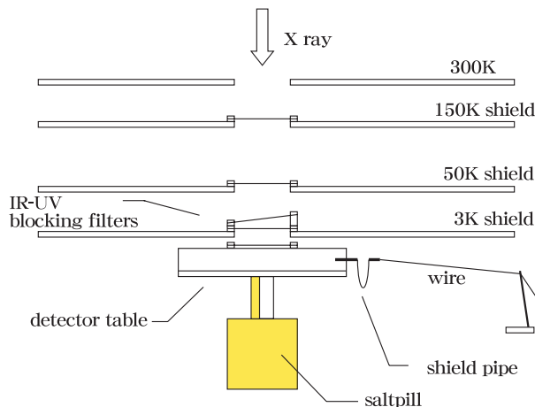
図 6.4: 入射窓の構造図。図にはないが 300K 部分は、ベリリウム窓か X 線ビームラインに直接コネクタでつながる。
