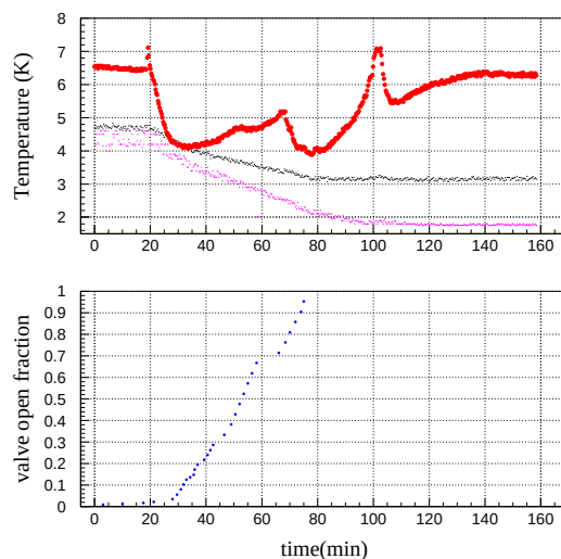
図 4.4: 液体ヘリウム減圧時の典型的な温度変化。He tank bottom で到達温度 1.7 K。ヒートスイッチは on。
