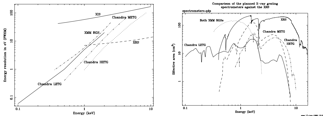
図 1.2: X 線分光器の性能比較。左: エネルギー分解能のエネルギー依存性 右: 有効面積のエネルギー依存性
