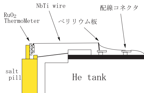
図 3.11: \text{RuO}_2 温度計 ( 1\text{k}\Omega ) の He 缶延長筒部分の配線
