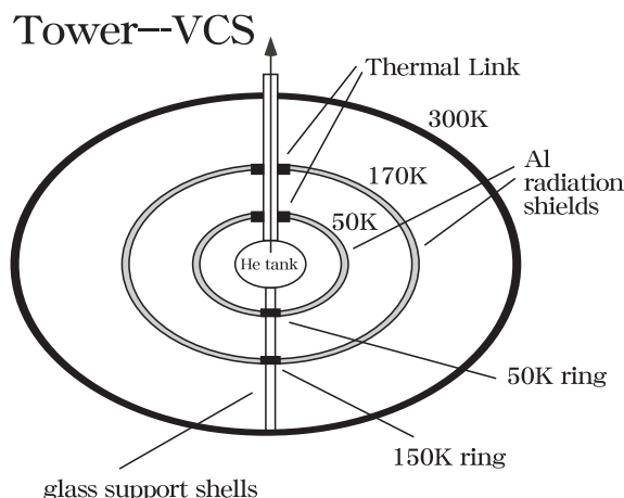
図 3.6: 本 ADR の VCS の構成図
