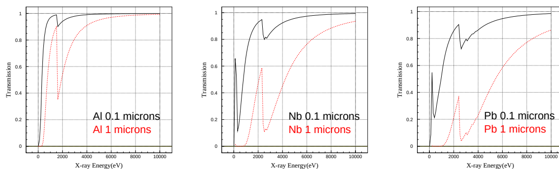
図 6.3: 各物質における X 線透過率。左から Al、Nb、Pb の場合。黒の実線は 0.1 \mu\text{m} 、赤の点線は 1 \mu\text{m} 。
