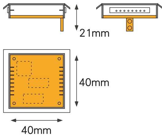
図 6.5: detector table プロトタイプの構造図
