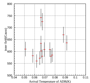
図 4.11: 断熱消磁試験結果の到達温度と内部磁場の関係。
