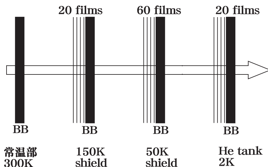
図 4.1: 実際の多層断熱の様子
