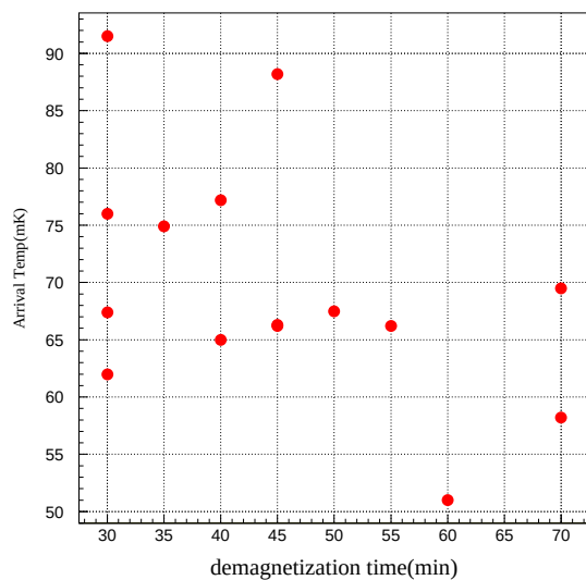
図 4.7: 主要な断熱消磁の際の磁化時間と内部磁場の関係。
