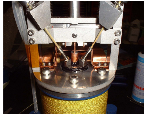
図 3.15: ヒートスイッチと saltpill の熱リンク
