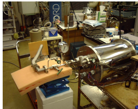
図 4.19: デュワーを横にした状態での断熱消磁試験の図
