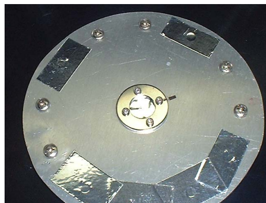
図 6.8: 3K shield の中央に導入した Blocking-Filter。0.1μm 厚の Al 蒸着された 9μm 厚マイラフィルムを使用。
