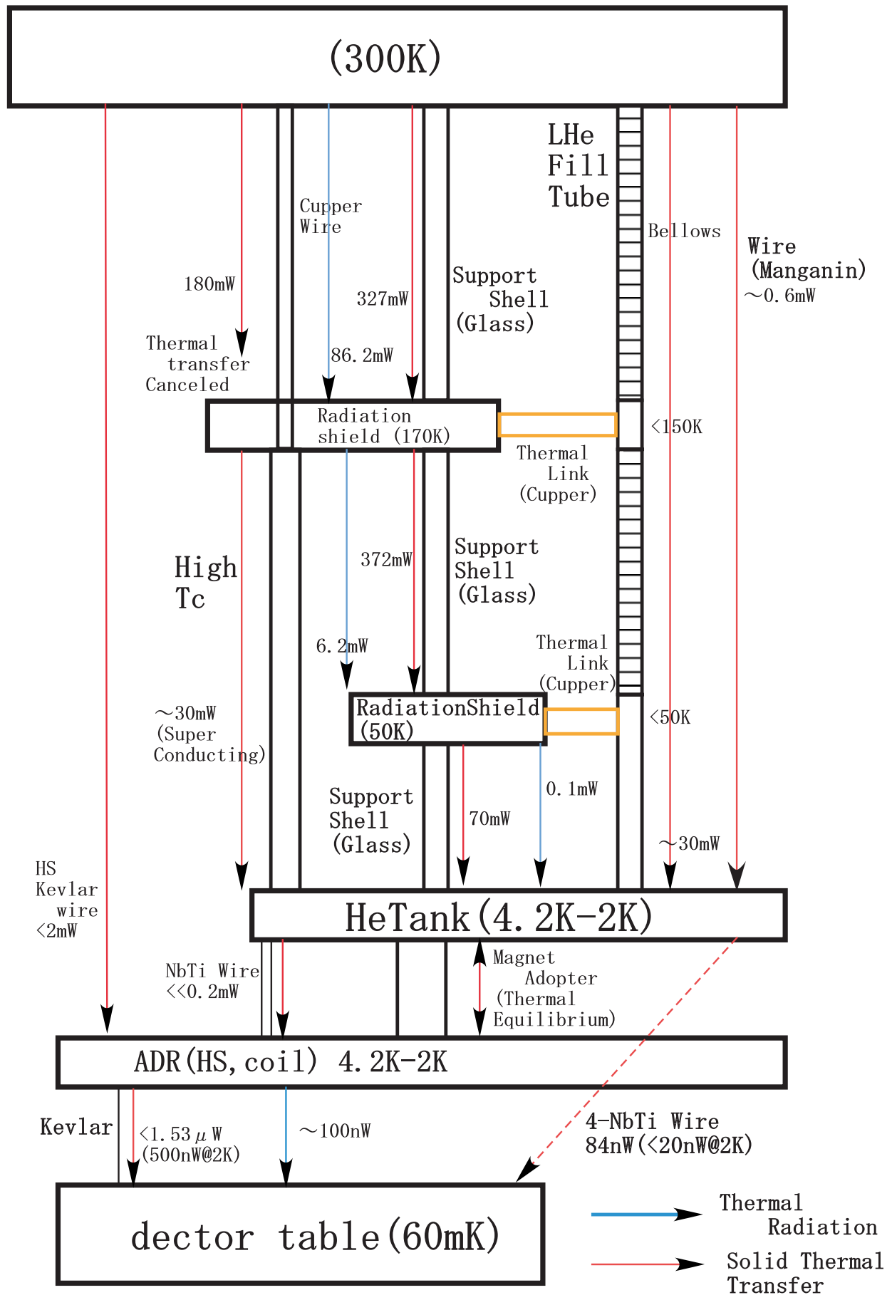
図 B.1: ADR デュワーの流入熱計算値
