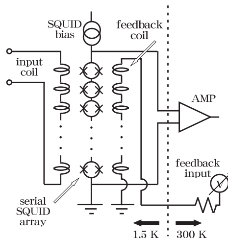
図 7.6: SSA AMP の回路図
