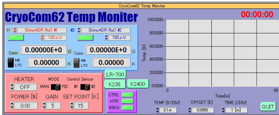
図 5.2: CryoCom62 panel(Lab Windows)
