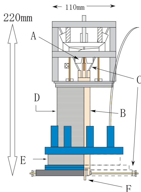
図 2.6: ADR 中心部の構造断面図。
