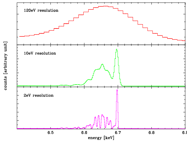
図 1.1: 温度 kT = 2 keV の光学的に薄いプラズマから放射される 6.7 keV の鉄輝線を、エネルギー分解能が 120 eV、10 eV、2 eV の検出器で観測した場合に得られるスペクトル (シミュレーション)
