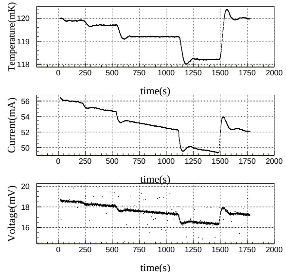
図 5.8: 設定温度を動かした時の変化の time scale。
