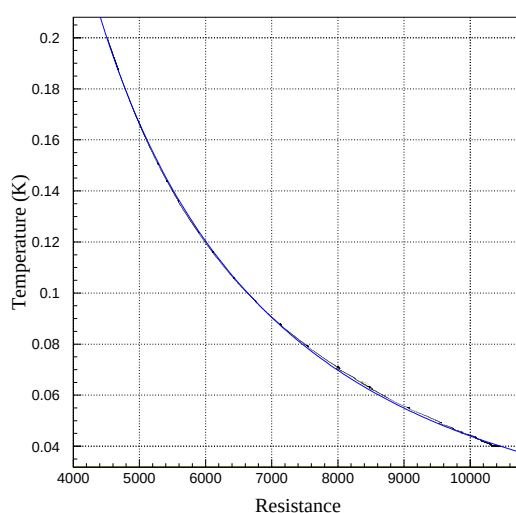
図 3.10: RuO 2 温度計の抵抗温度特性
