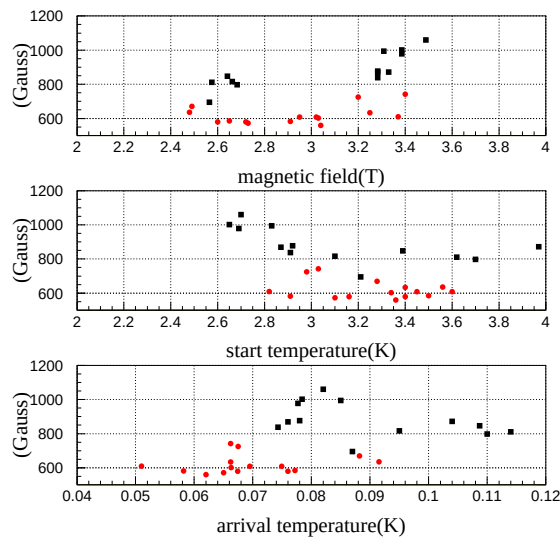
図 6.1: 左 : detector table プロトタイプ導入前と導入後の冷却試験の比較。黒 (四角) : 導入前。赤 (丸) : 導入後
