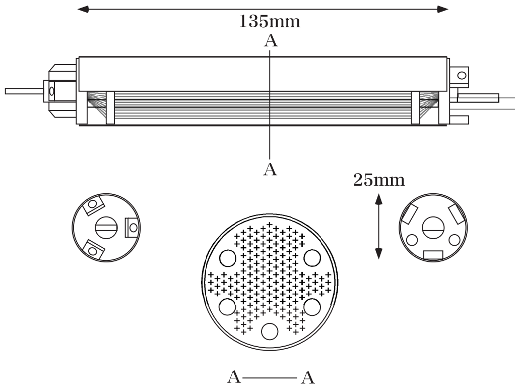
図 3.16: ADR salpill 2 号機の構造図
