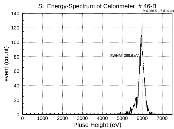
図 5.53: シリコンイベントの X 線スペクトル
