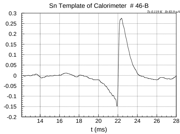
図 5.49: スズイベントの最適フィルタテンプレート
