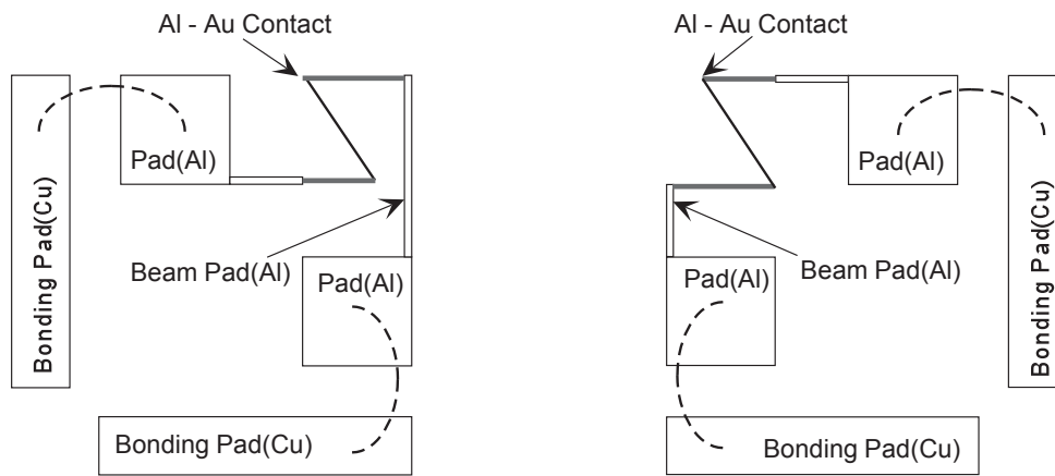
図 4.4: カロリメータのボンディングの様子
