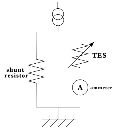
図 2.10: 疑似的な定電圧回路
