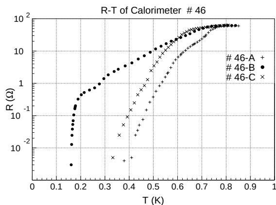
図 4.7: カロリメータ #46 の R-T 特性
