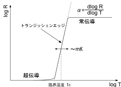
図 2.1: トランジションエッジ
