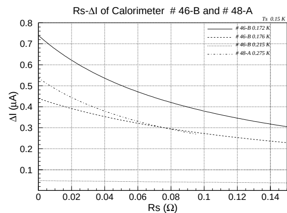
図 4.32: シャント抵抗と電流変化の関係
