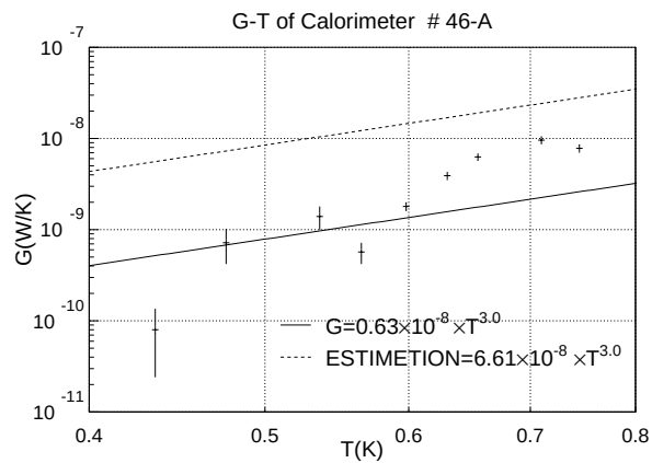
図 4.13: カロリメータ #46-A の G-T 特性
