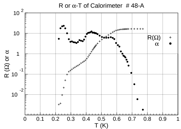
図 4.12: カロリメータ #48-A の R-T 特性と \alpha
