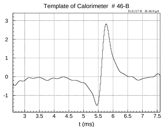
図 5.21: 最適フィルタテンプレート
