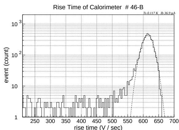
図 5.17: RT の分布
