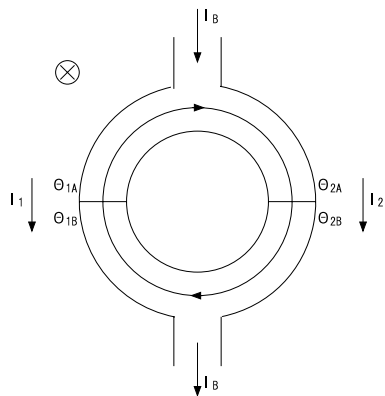
図 2.7: dc-SQUID
