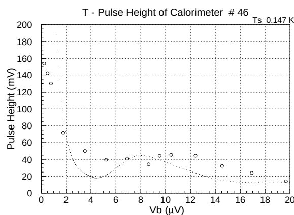
図 5.40: バイアス電圧とパルスハイトの関係
