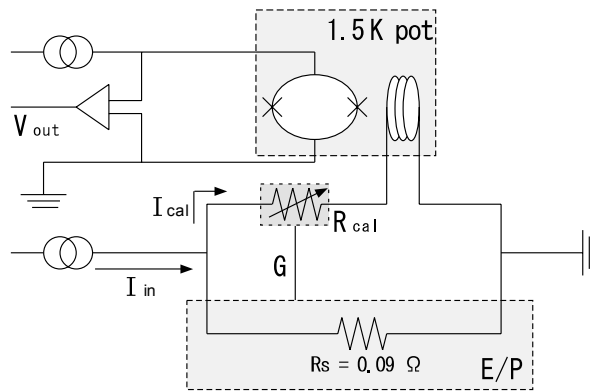
図 5.4: 動特性を測定する回路構成の模式図
