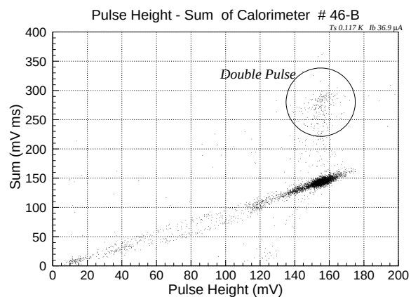
図 5.13: PH と SUM の関係
