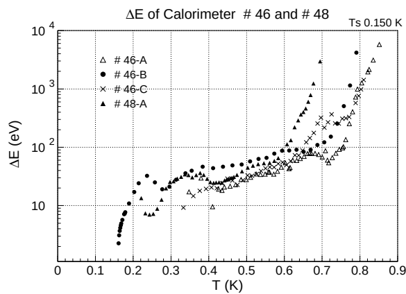
図 4.17: 動作点温度に対するカロリメータのエネルギー分解能
