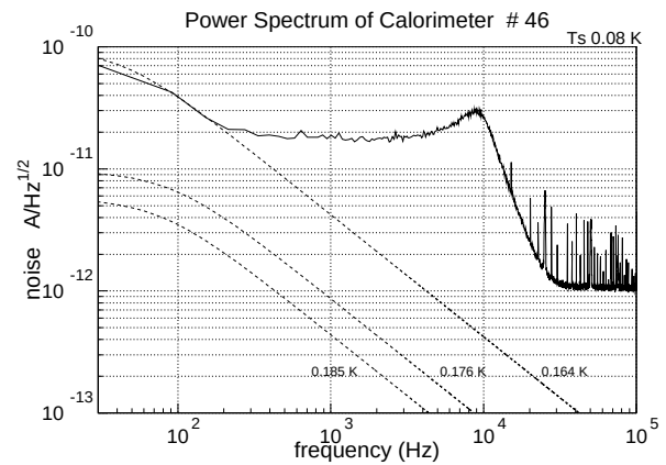
図 5.61: フォノンノイズと動作温度の関係
