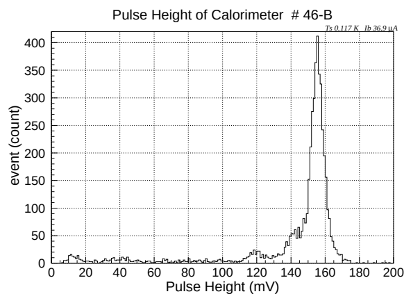
図 5.12: PH の分布
