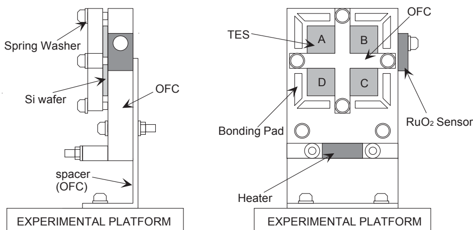
図 4.3: カロリメータのサンプルステージ
