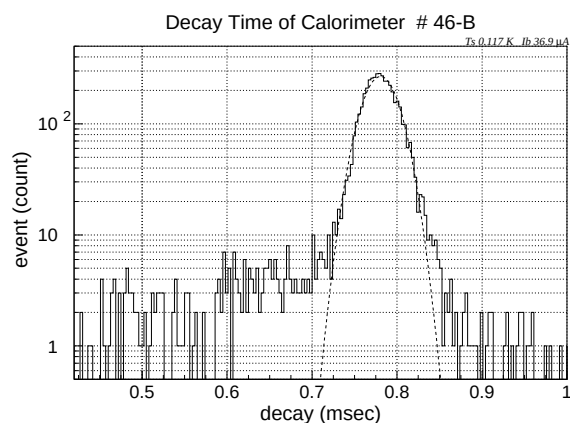
図 5.16: -1/\text{DECAY} の分布
