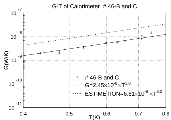
図 4.16: カロリメータ #46-B, C の G-T 特性
