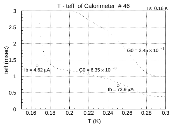
図 5.26: 有効時定数
