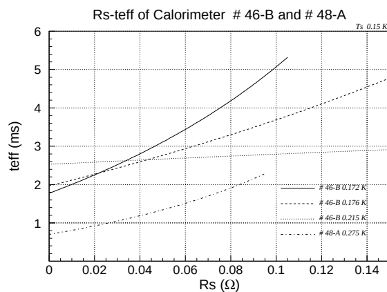
図 4.31: シャント抵抗と有効時定数の関係
