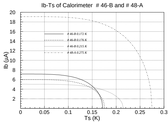
図 4.25: 熱浴の温度とバイアス電流の関係
