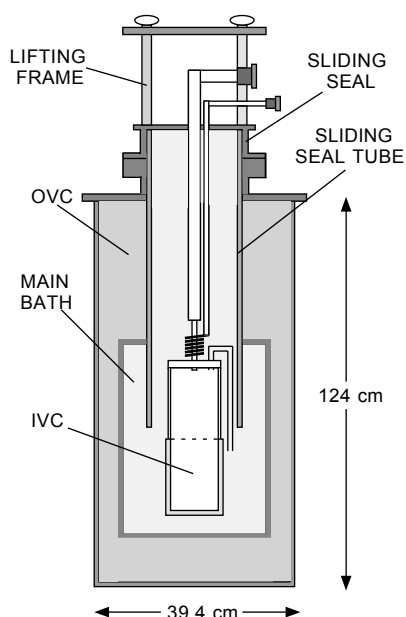
図 3.1: 希釈冷凍機のユニット
