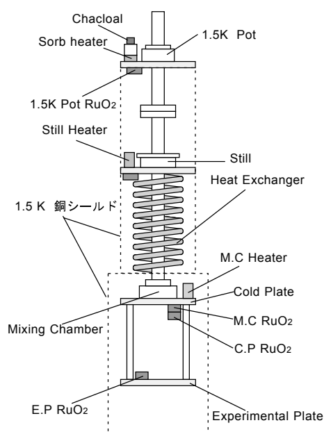
図 3.2: IVC 内部の主要な器官
