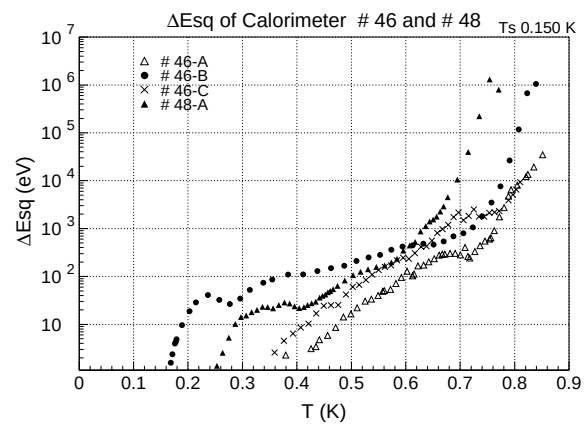
図 4.18: 動作温度に対する SQUID のエネルギー分解能
