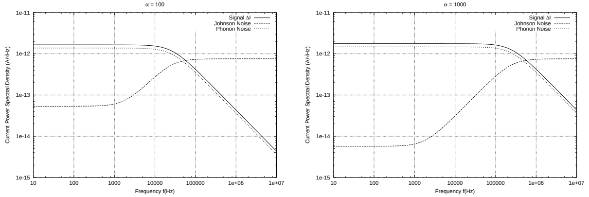
図 2.5: ノイズ電流 power spectral density 左: \alpha = 100 右: \alpha = 1000 低い周波数では、電熱フィードバックによってジョンソンノイズが抑制される。
