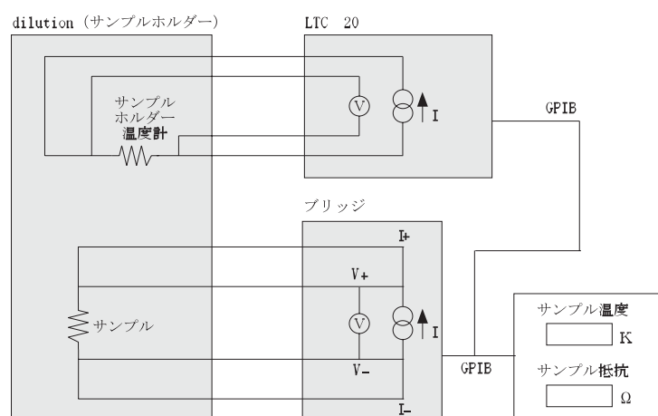
図 4.5: 測定系の配線図
