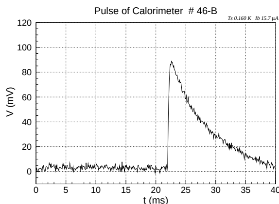
図 5.30: 典型的な X線パルス
