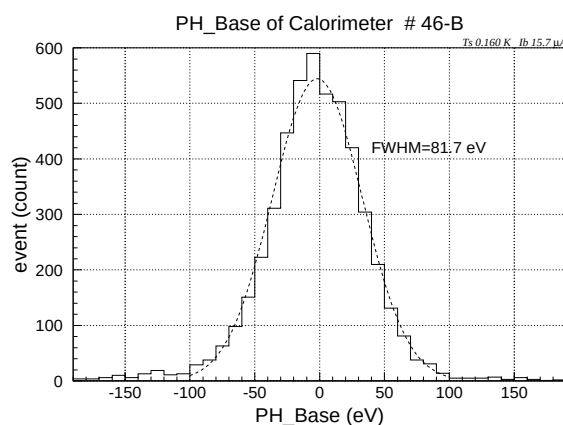
図 5.35: ベースラインのノイズによる寄与
