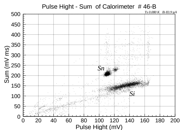
図 5.44: PH と SUM の関係
