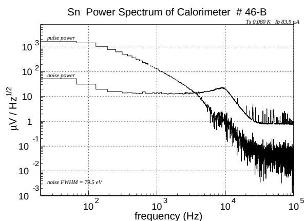
図 5.47: スズイベントのノイズとパルスのパワースペクトル
