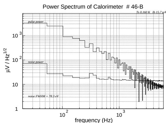
図 5.32: ノイズとパルスのパワースペクトル
