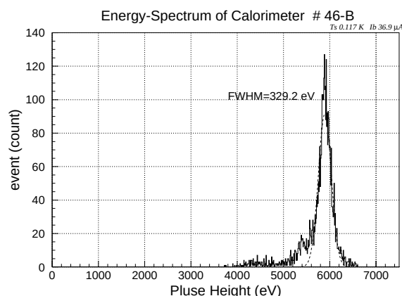
図 5.22: X 線スペクトル
