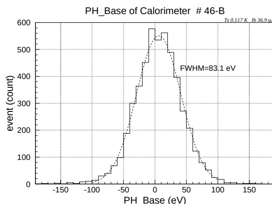
図 5.23: ベースラインのノイズによる寄与
