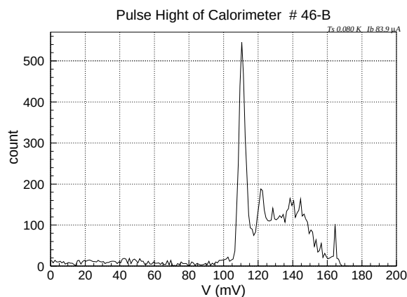
図 5.43: PH とカウント数
