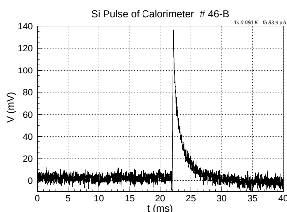
図 5.42: Si イベントの典型的な X 線パルス
