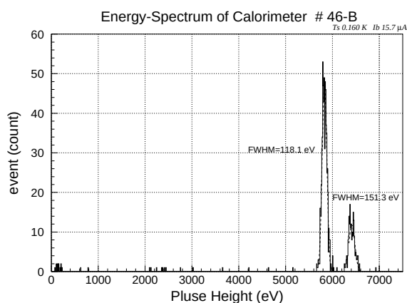
図 5.34: X 線スペクトル
