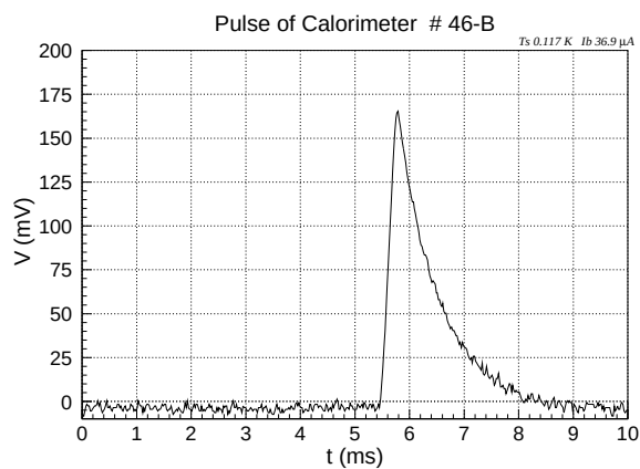
図 5.10: 典型的な X 線パルス
