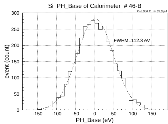
図 5.54: シリコンイベントのベースラインのノイズの寄与
