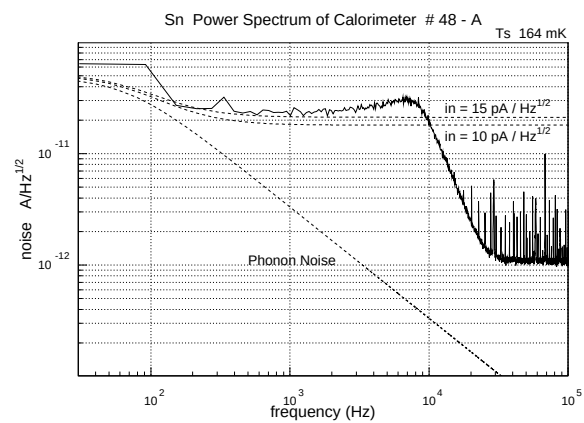
図 5.69: ベースラインのパワースペクトル
