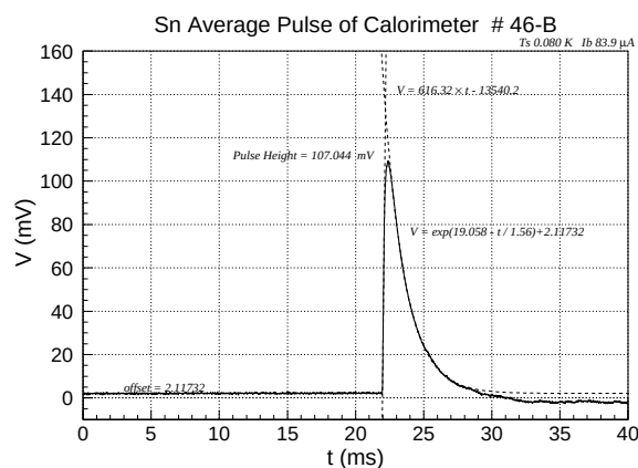
図 5.45: スズイベントの平均パルス
