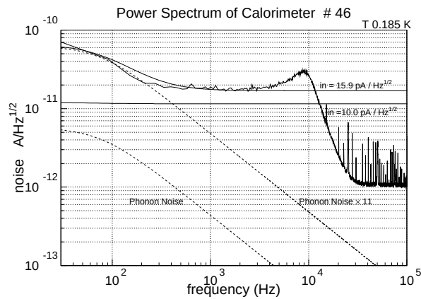
図 5.60: ベースラインのパワースペクトル
