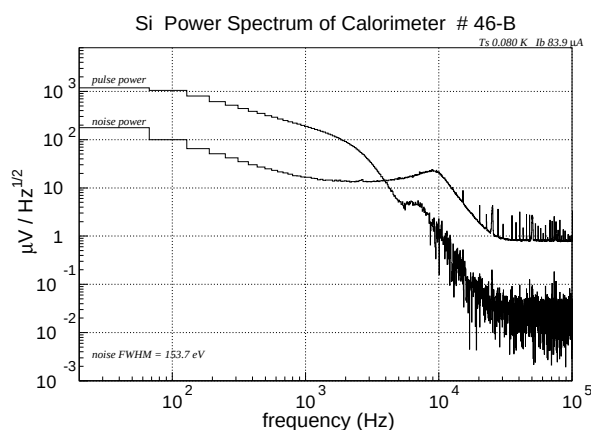
図 5.48: シリコンイベントのノイズとパルスのパワースペクトル
