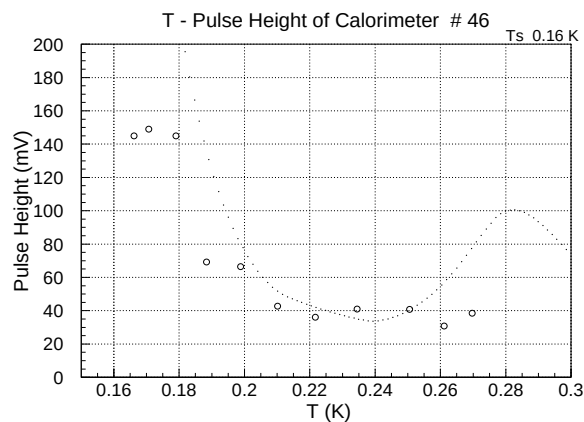
図 5.25: 熱浴の温度が 0.16 K におけるパルスの最大値と見積もりとの比較
