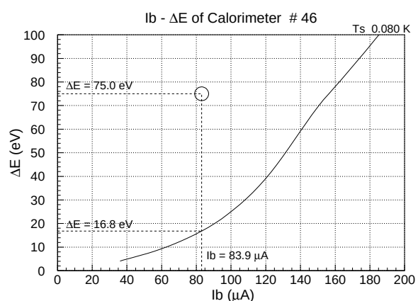
図 5.56: バイアス電流とエネルギー分解能の関係
