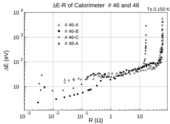
図 4.19: 動作点抵抗に対するエネルギー分解能
