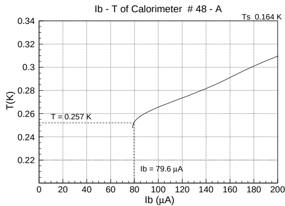
図 5.68: バイアス電流と動作温度の関係
