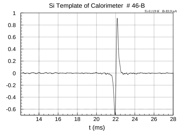
図 5.50: シリコンイベントの最適フィルタテンプレート
