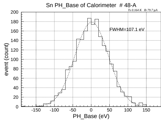
図 5.67: スズイベントのベースラインによるノイズの寄与
