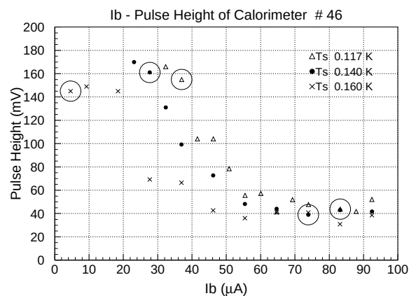
図 5.9: バイアス電流とパルスハイトとの関係
