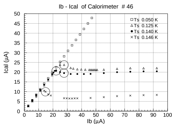
図 5.28: バイアス電流 I_b とカロリメータに流れる電流 I_{\text{cal}} の関係
