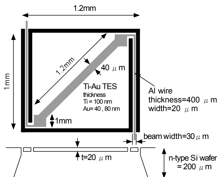
図 4.2: カロリメータの構造の模式図
