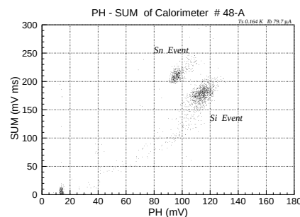
図 5.65: PH と SUM の関係
