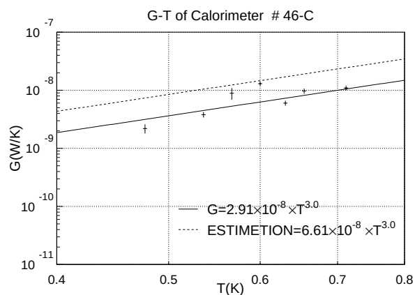
図 4.15: カロリメータ #46-C の G-T 特性
