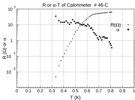
図 4.11: カロリメータ #46-C の R-T 特性と \alpha
