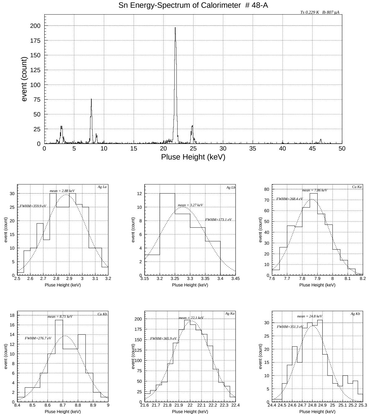
図 5.71: ^{109}\text{Cd} を照射して取得した X 線スペクトル
