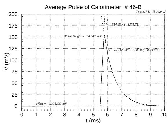
図 5.19: 平均パルス
