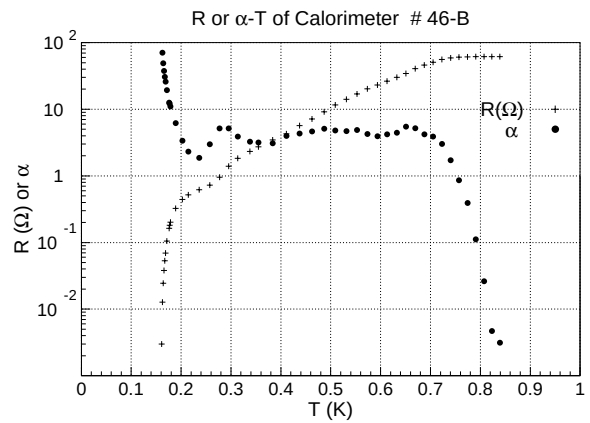
図 4.10: カロリメータ #46-B の R-T 特性と \alpha
