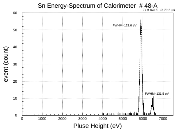
図 5.66: スズイベントの X 線スペクトル
