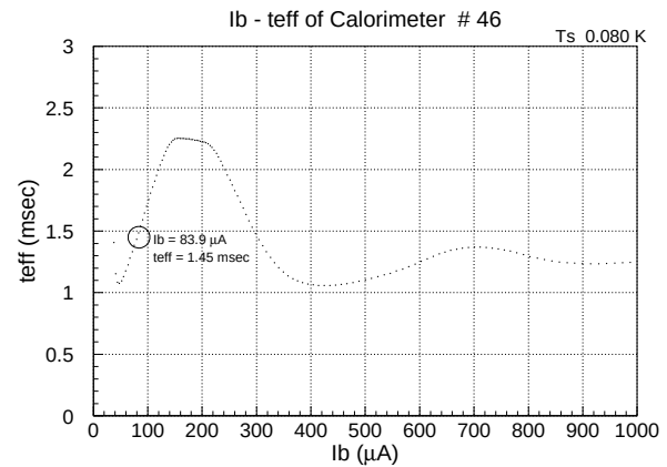
図 5.59: バイアス電流と有効時定数の関係
