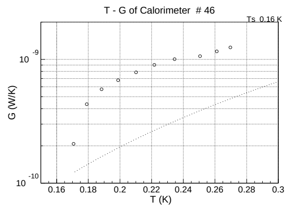
図 5.7: 温度と熱伝導度の関係
