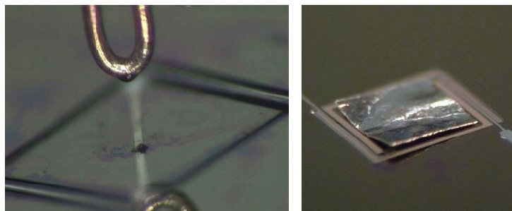
図 5.27: 吸収体取り付けの様子
