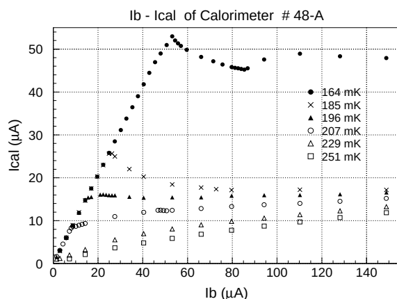
図 5.63: バイアス電流とカロリメータに流れる電流の関係
