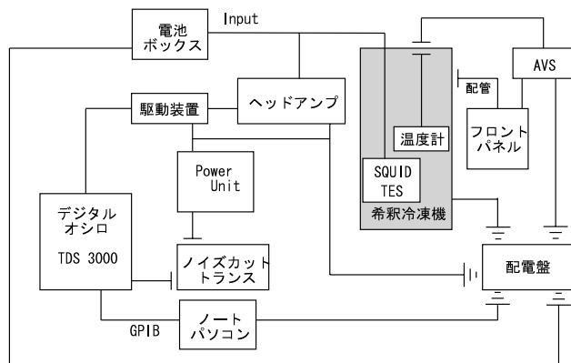
図 5.2: 測定系のグランドまわり
