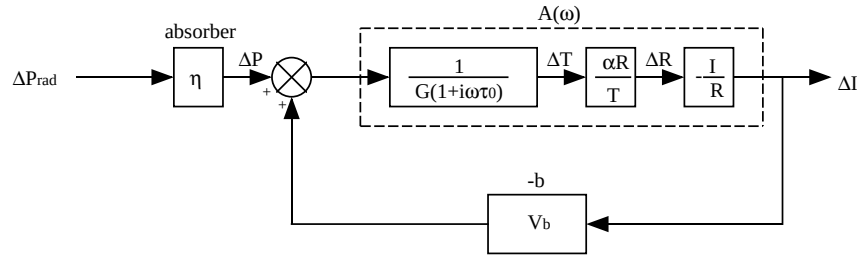
図 2.3: 電熱フィードバックの回路の模式図
