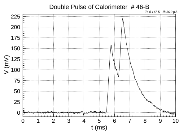
図 5.14: ダブルパルス
