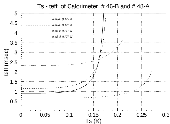
図 4.27: 熱浴の温度と有効時定数の関係
