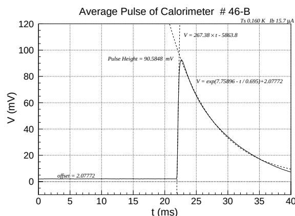
図 5.31: 平均パルス
