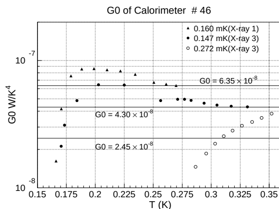
図 5.39: G_0 のプロット
