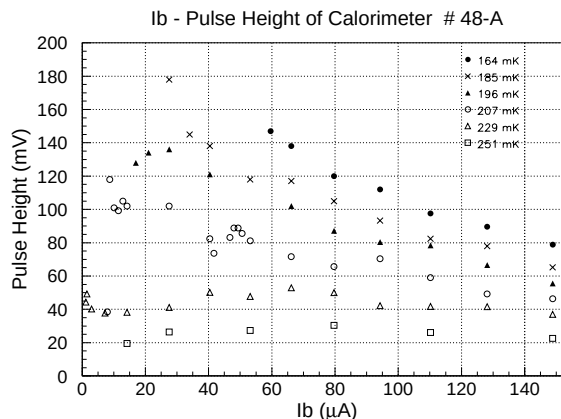
図 5.64: バイアス電流と X 線パルスの最大値との関係
