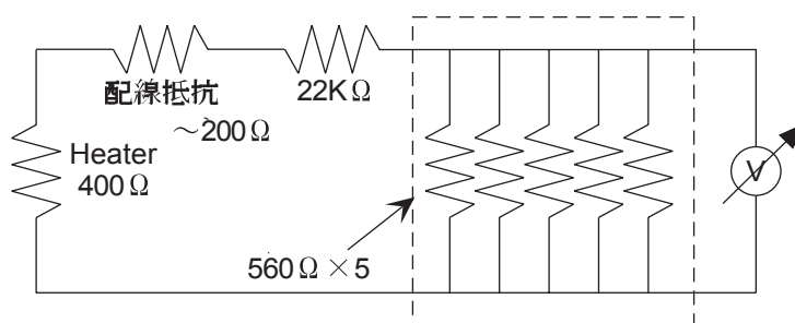
図 4.6: ヒータの分流回路
