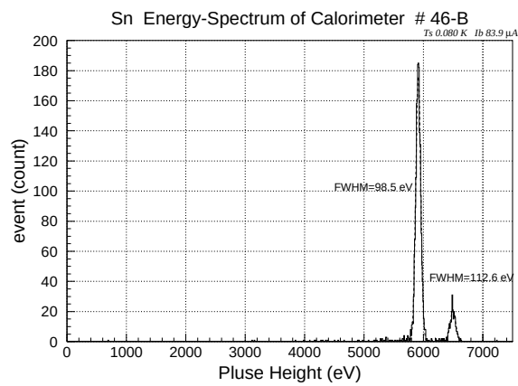
図 5.51: スズイベントの X 線スペクトル
