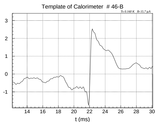
図 5.33: パルスのテンプレート
