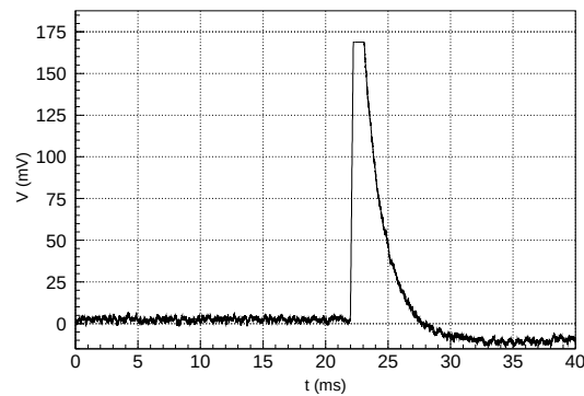
図 5.72: 46.4 keV 付近にある X 線イベント
