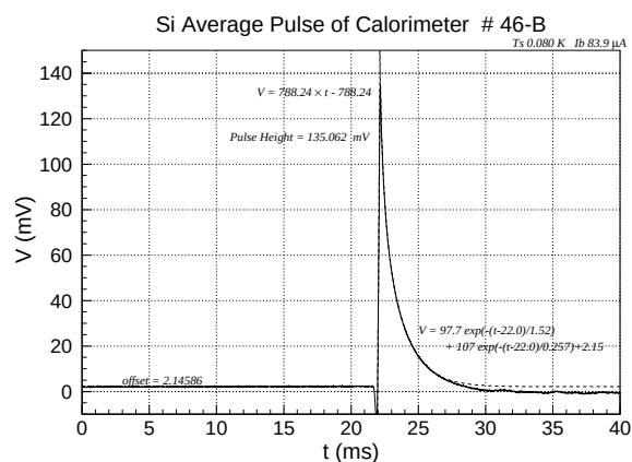
図 5.46: シリコンイベントの平均パルス
