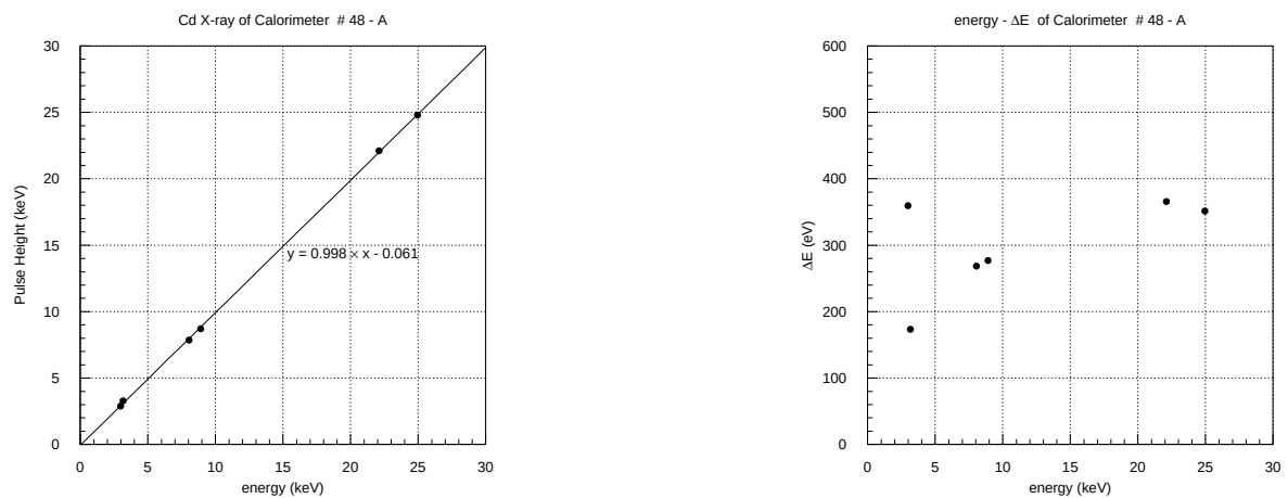
図 5.73: 実測との比較
