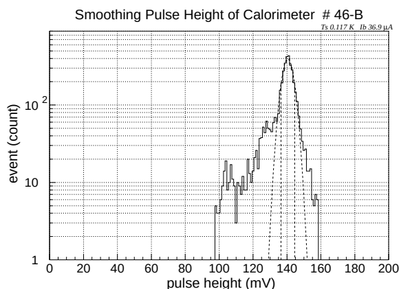
図 5.18: スムージングしたときのパルス高の分布
