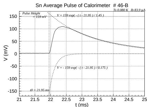
図 5.57: 二つの指数関数でフィットした平均パルス
