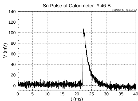
図 5.41: Sn イベントの典型的な X 線パルス
