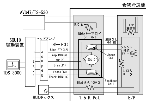
図 5.1: X 線照射実験の回路図
