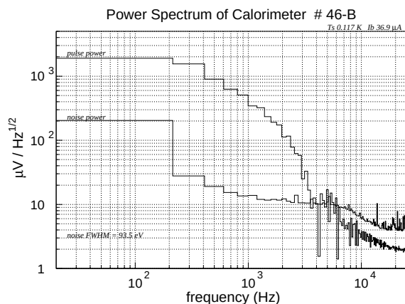
図 5.20: ノイズとパルスのパワースペクトル
