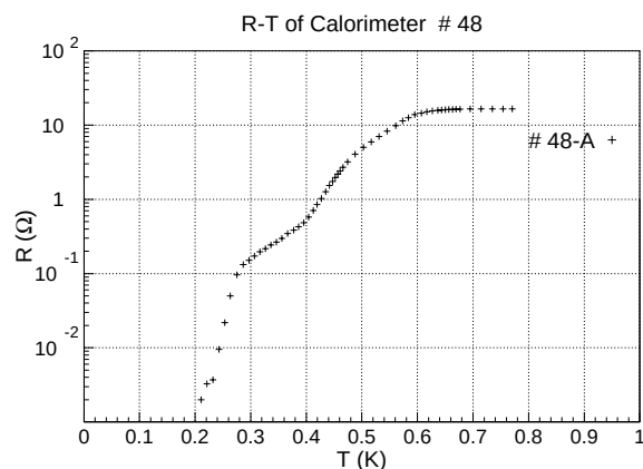
図 4.8: カロリメータ #48 の R-T 特性
