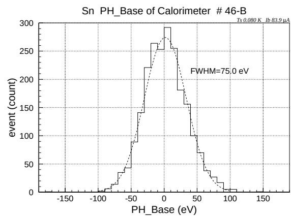
図 5.52: スズイベントのベースラインによるノイズの寄与
