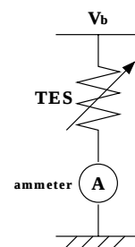
図 2.2: 定電圧バイアス
