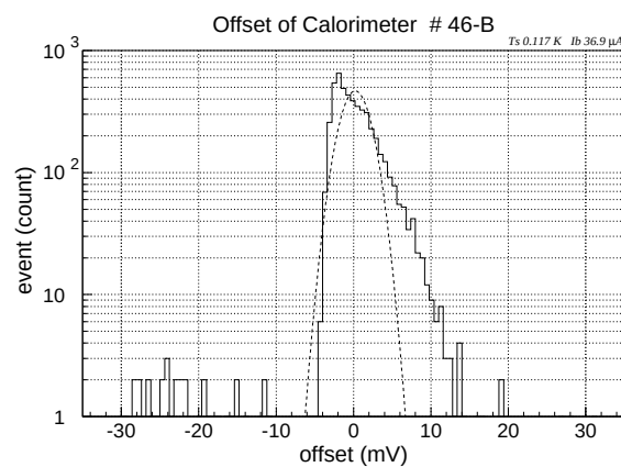
図 5.15: OFFSET の分布
