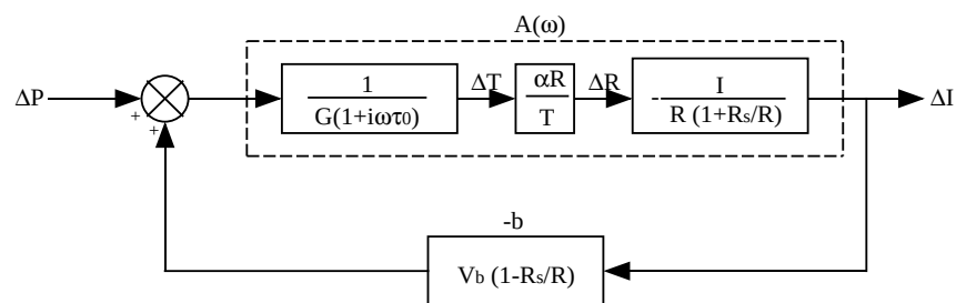
図 2.11: 疑似的な定電圧バイアスを考慮して補正したダイアグラム
