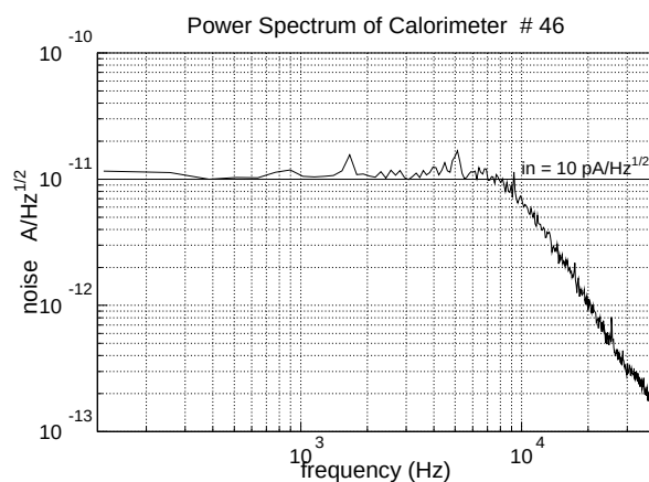
図 3.4: SQUID のノイズスペクトル
