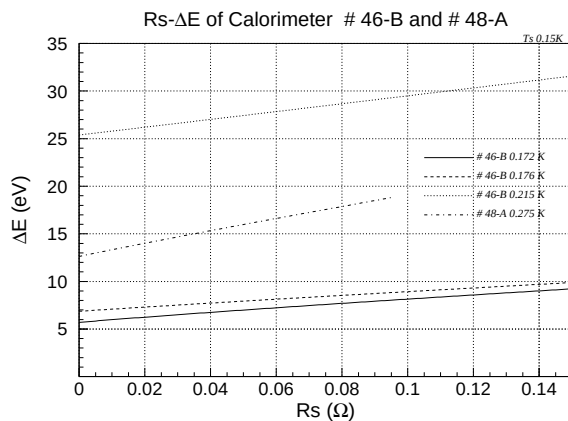
図 4.29: シャント抵抗とカロリメータのエネルギー分解能の関係
