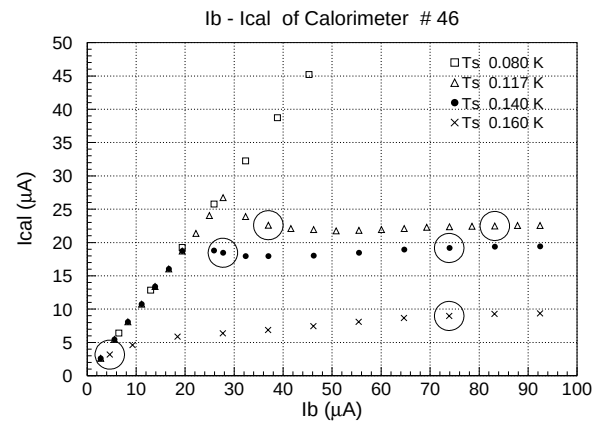
図 5.5: バイアス電流 I_b とカロリメータに流れる電流 I_{cal} の関係
