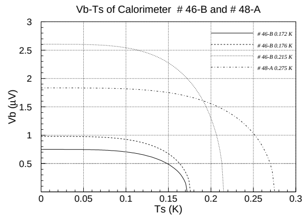
図 4.26: 熱浴の温度とバイアス電圧の関係
