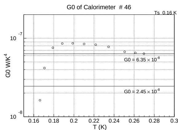
図 5.24: G_0 のプロット
