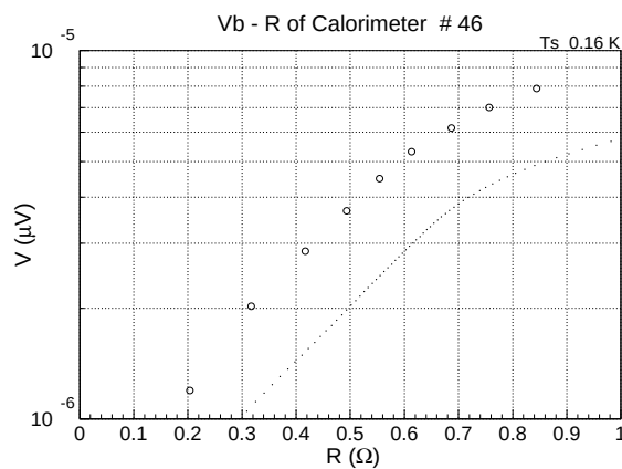
図 5.6: 抵抗とバイアス電圧の関係
