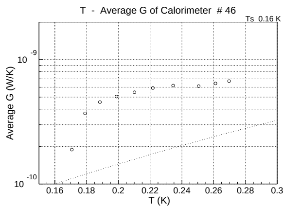
図 5.8: 温度と平均の熱伝導度の関係
