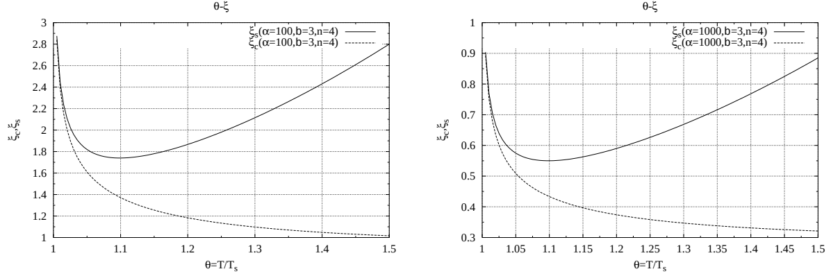
図 2.6: \xi と \theta = T/T_s の関係左: \alpha = 100 右: \alpha = 1000 .
