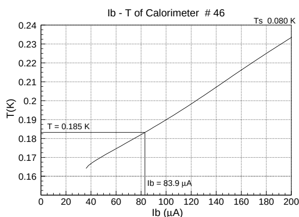
図 5.55: バイアス電流と動作温度の関係
