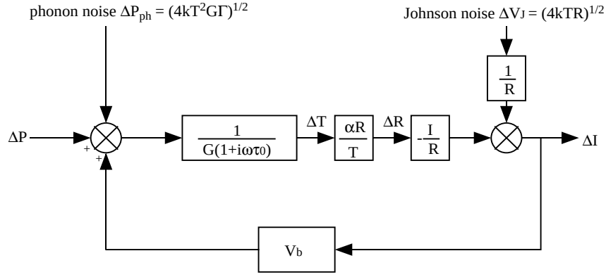
図 2.4: ノイズも含めたダイアグラム
