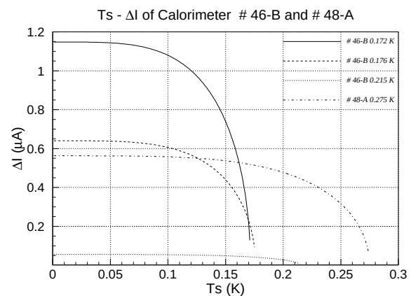
図 4.28: 熱浴の温度と電流変化の関係
