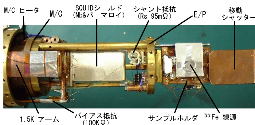
図 5.3: 希釈冷凍機の組み込みの写真
