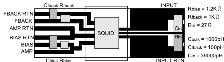
図 3.3: 使用した SQUID 素子。基板はガラスエポキシ。
