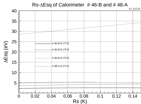
図 4.30: シャント抵抗と SQUID のエネルギー分解能の関係
