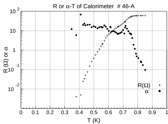
図 4.9: カロリメータ #46-A の R-T 特性と \alpha
