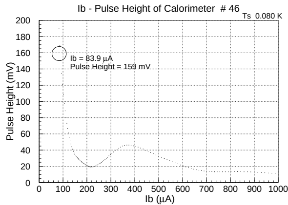
図 5.58: バイアス電流とパルスハイトの関係
